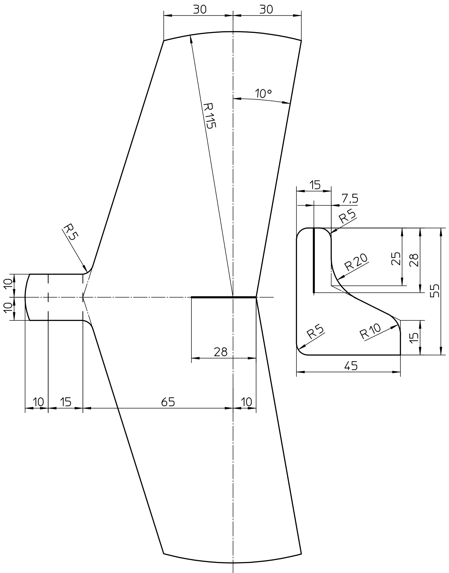
Papierflugzeug PTT-Papptellertaube D. M. Krone www.papierfliegerei.de
